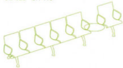
S6G12 6 seater + 1 table OH 800 OW 3790 OD 620 SH 415
