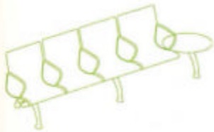
S4G11 4 seater + 1 table OH 800 OW 2665 OD 620 SH 415
