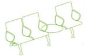
S3G11 3 seater + 1 table OH 800 OW 2120 OD 620 SH 415
