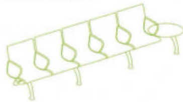
S5G11 5 seater + 1 table OH 800 OW 3210 OD 620 SH 415
